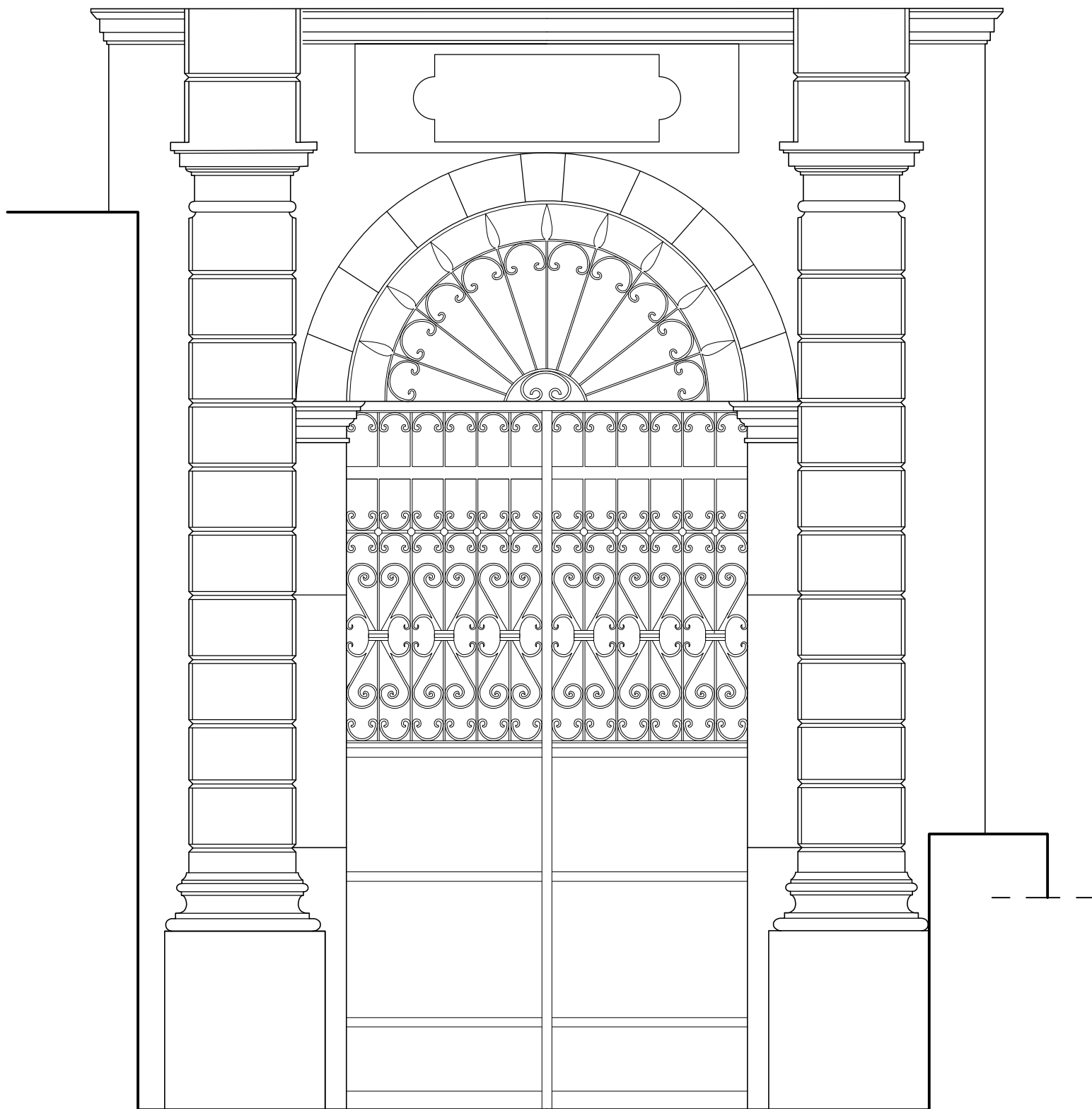
ΕΞΩΤΕΡΙΚΗ ΟΨΗ
