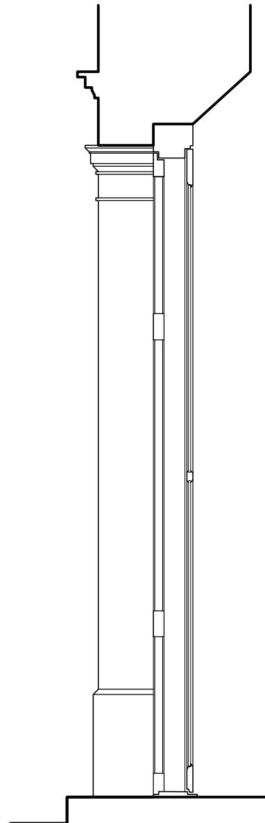
ΤΟΜΗ
