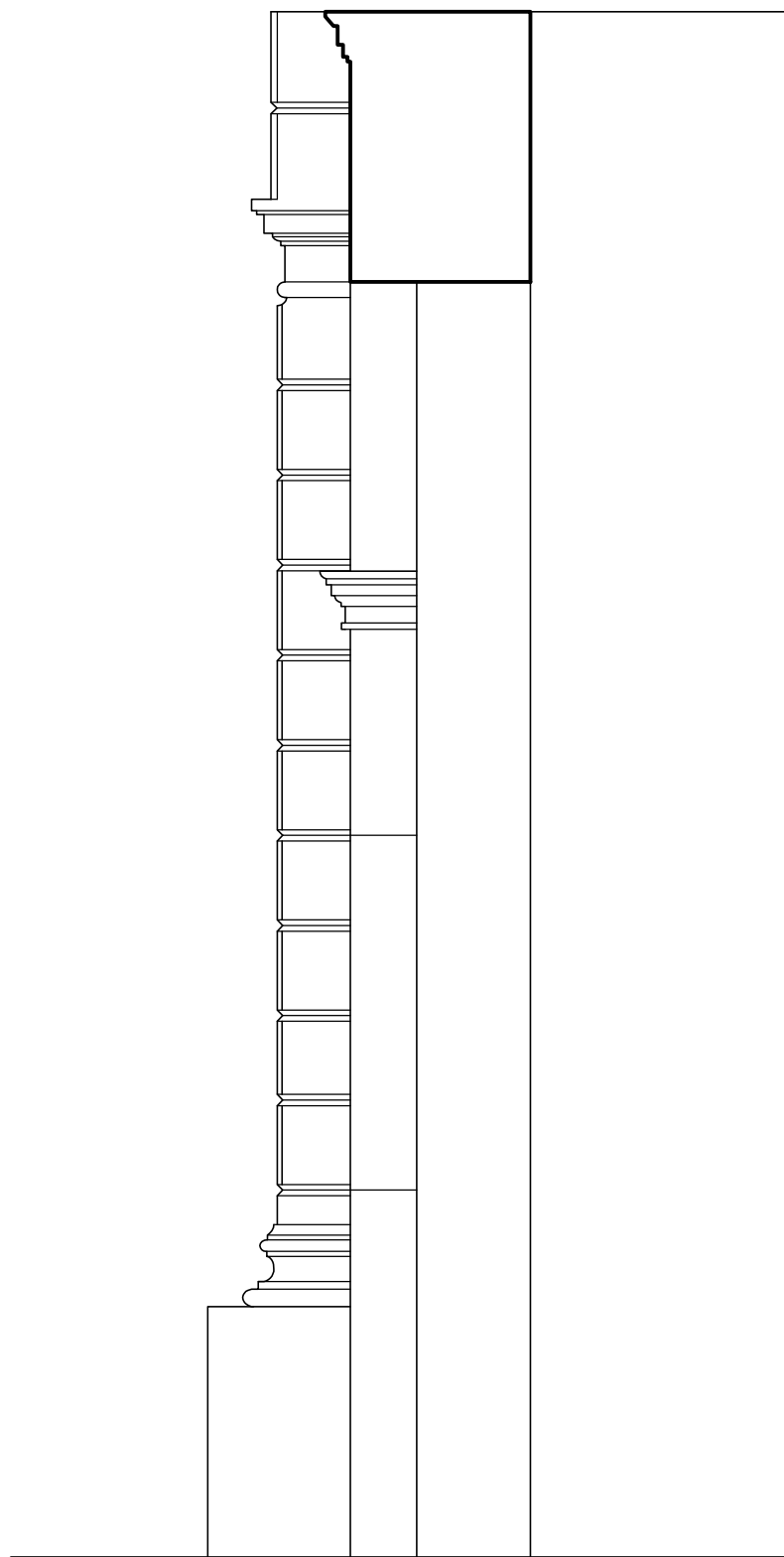
ΤΟΜΗ
