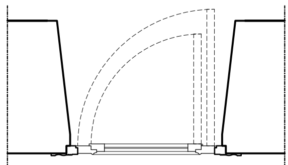
ΚΑΤΟΨΗ
